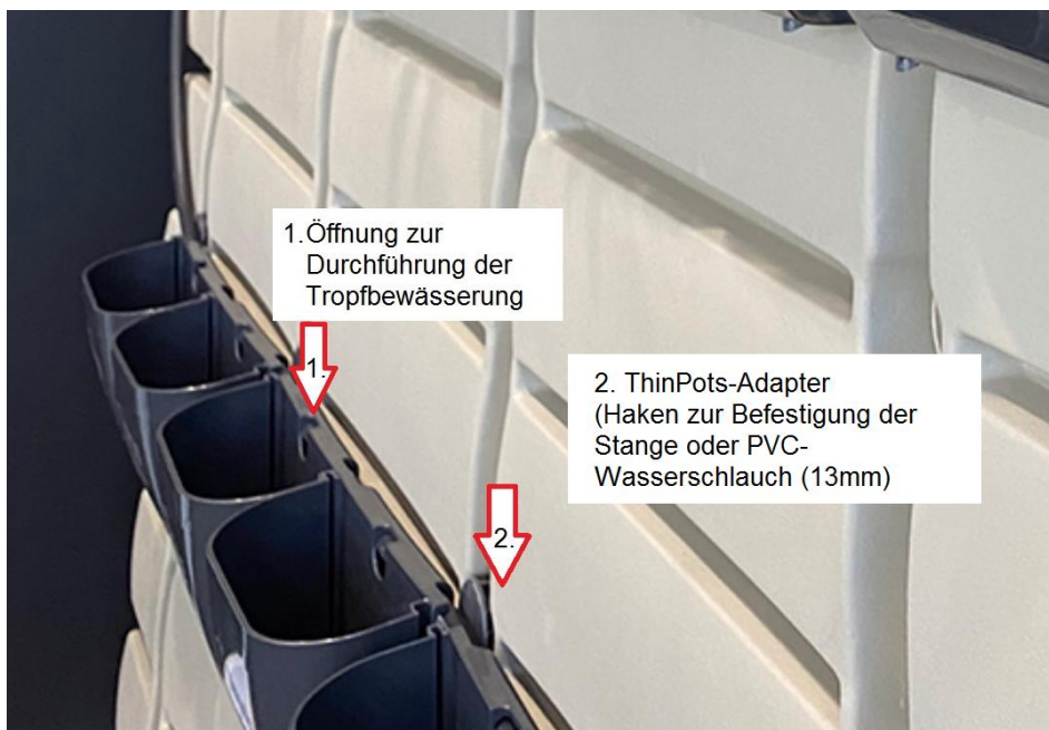
Bild: Montage ThinPots und Anschlussmöglichkeiten einer Tropfbewässerung
