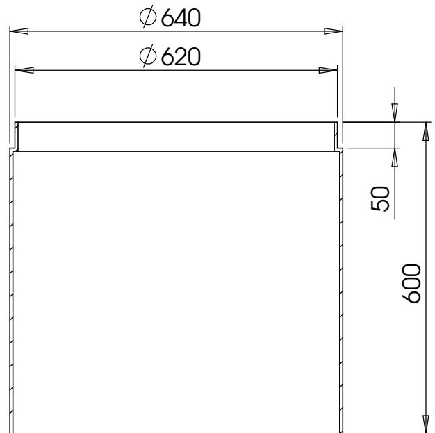
SCHNITT A-A MAßSTAB 1 : 10
