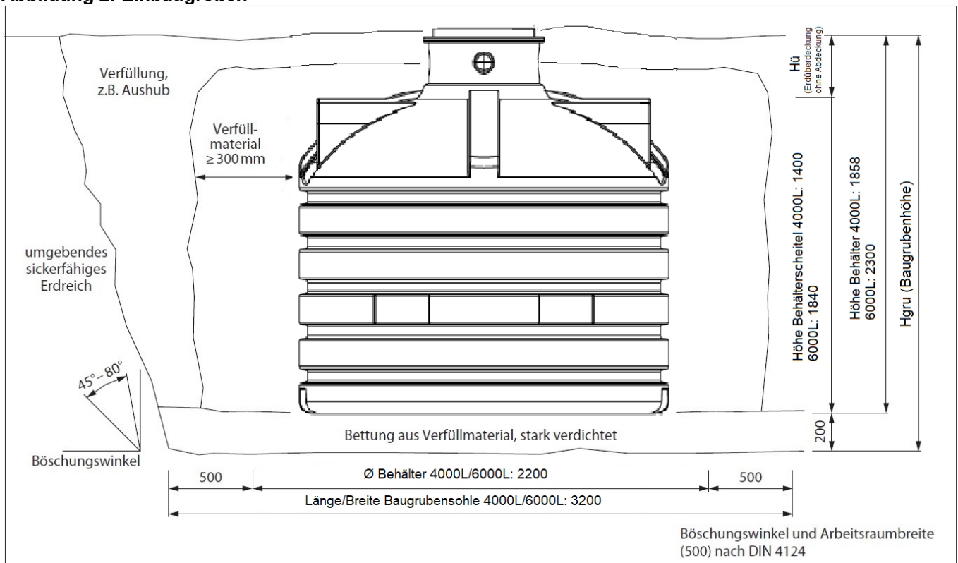
Abbildung 2: Einbaugrößen
