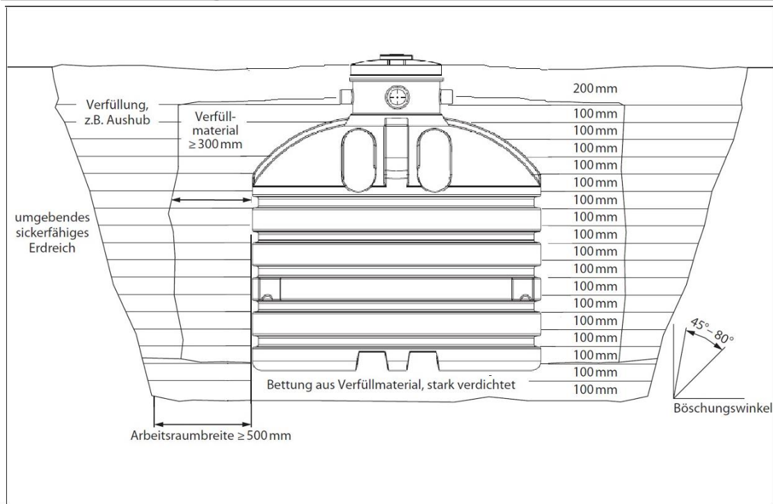
Abbildung 4: Ausführung des Einbaus am Beispiel eines Oasis 6000 L Erdtanks mit Tankabdeckung Basic
