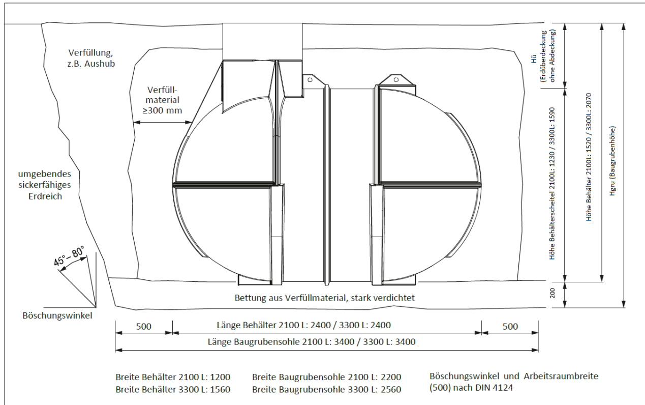
Abbildung 2: Einbaugrößen
