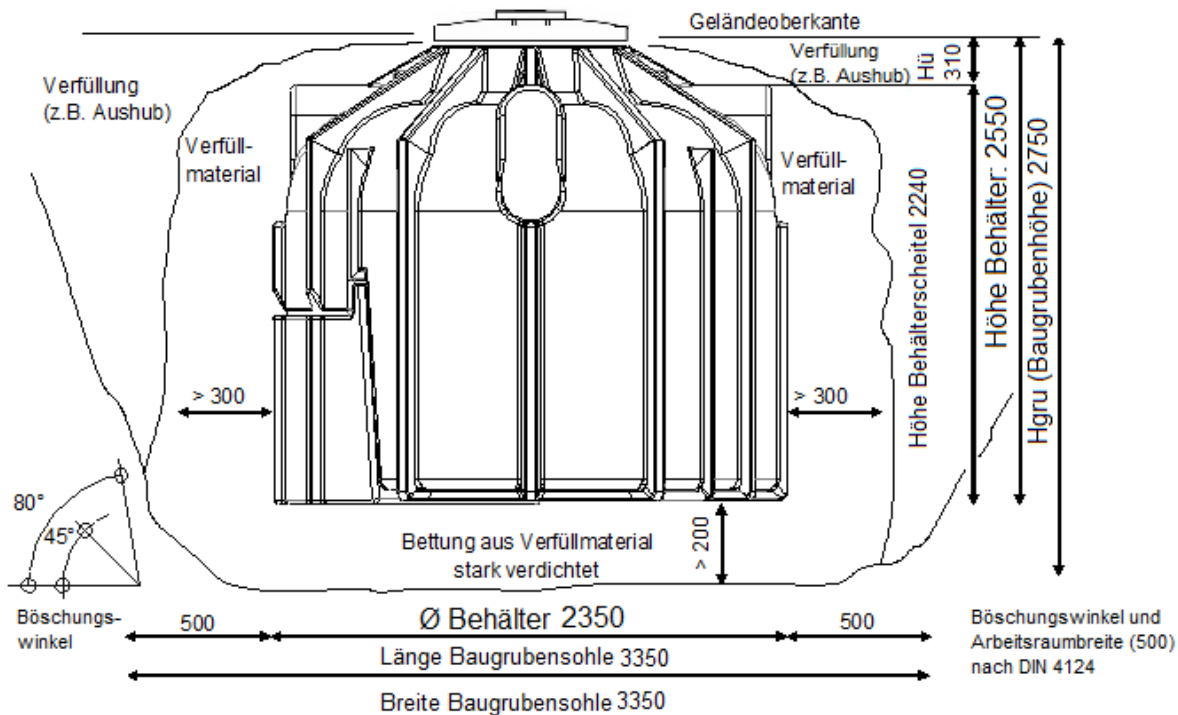
Abbildung 2: Einbaugrößen
