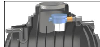
Abb. 1: Montierter Filter & Siphon
