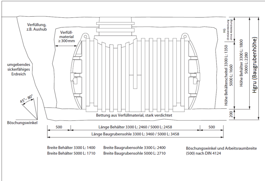
Abbildung 2: Einbaugrößen
